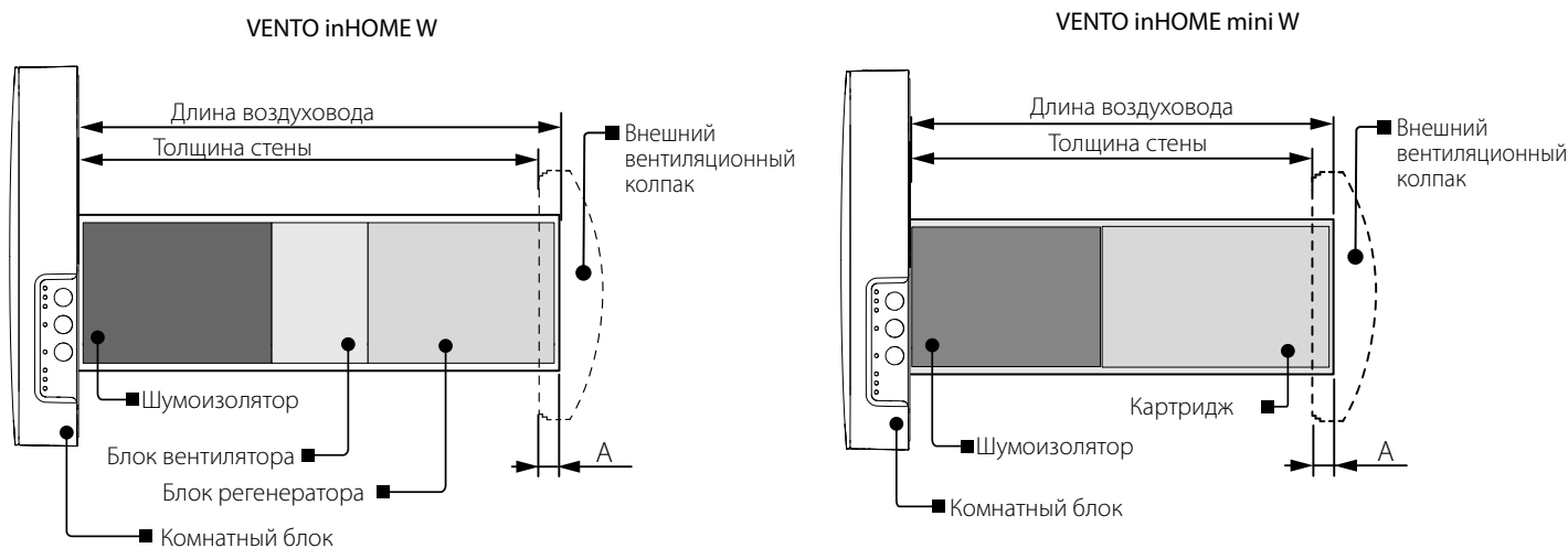
Схема расположения узлов проветривателя внутри стены
