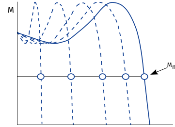
График крутящего момента при пуске от ПЧ
