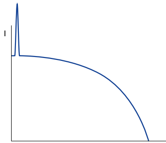
График тока при прямом пуске
