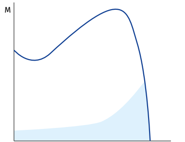
График крутящего момента при прямом пуске
