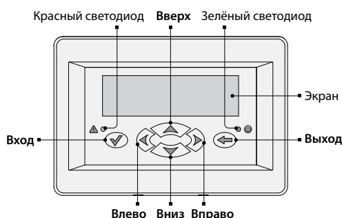
Рис. 2 Функции кнопок панели управления
