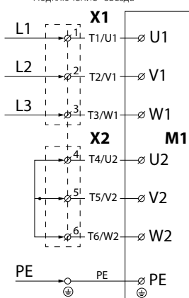
Схема подключения к электросети для вентилятора с односкоростным электродвигателем
