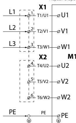
Схема подключения к электросети для вентилятора с двухскоростным электродвигателем
