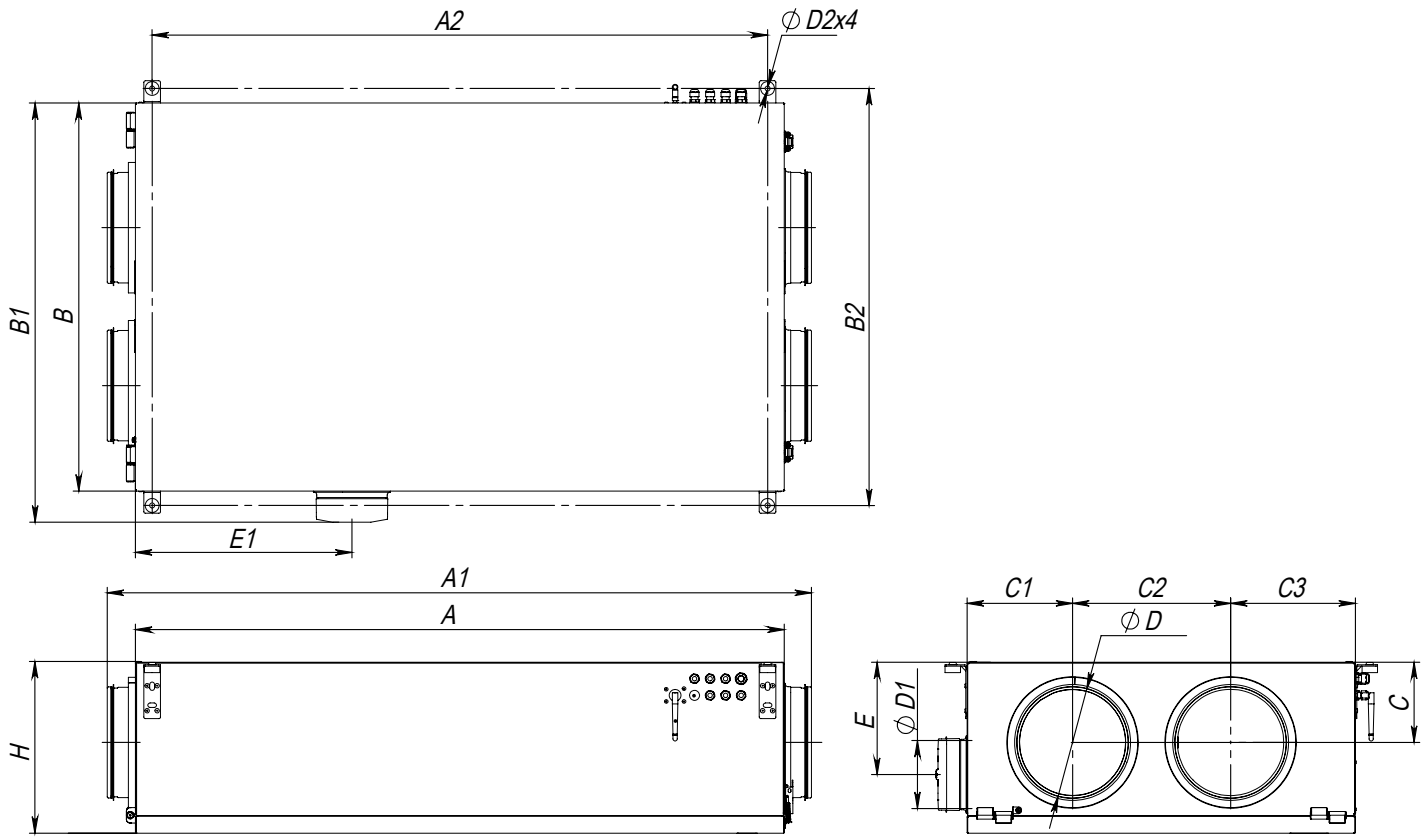
KOMFORT Roto EC D(E) 351
